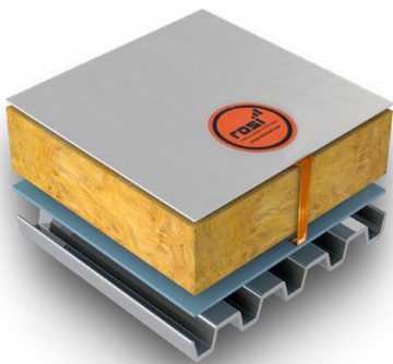
Einbaubeispiel bei frei bewitterten Dachflächen
