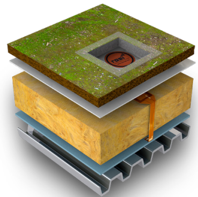
Einbaubeispiel bei aufgelasteten Flächen
