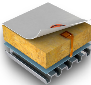
Platzierung des Sensors und der Sensorantenne
